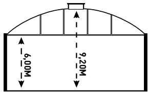
COUPE
